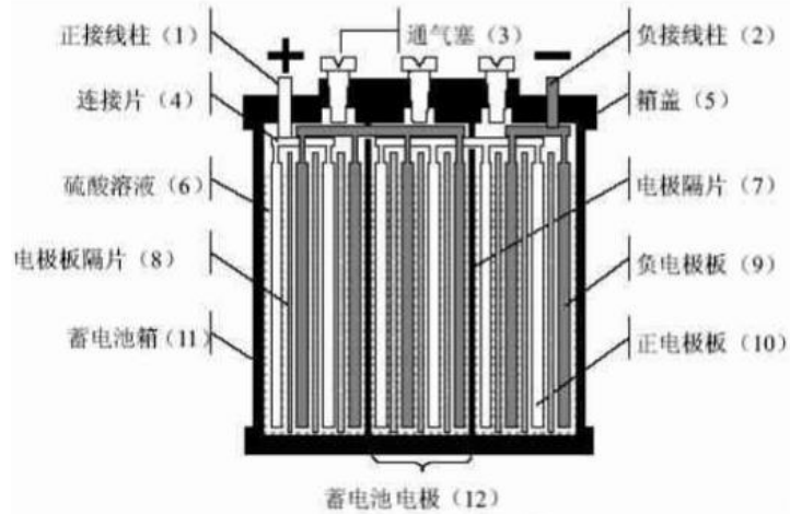
图5-2 铅酸蓄电池典型结构图
