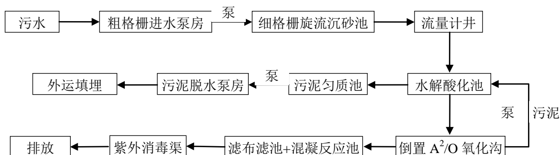
图 7-1 沭阳南方水务有限公司（原沭阳城南污水处理厂）工艺流程图
